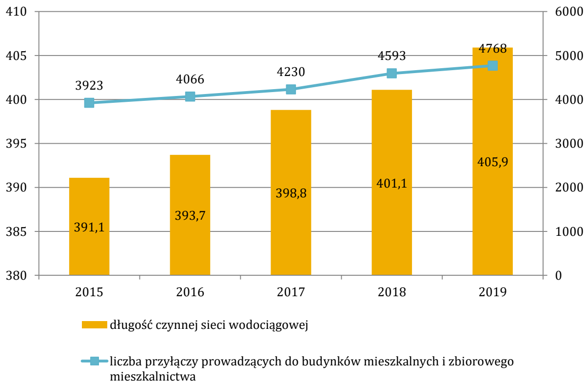
Wykres 16. Długości czynnej sieci wodociągowej [km] oraz liczba przyłączy w gminie Chełmiec w latach 2015-2019
