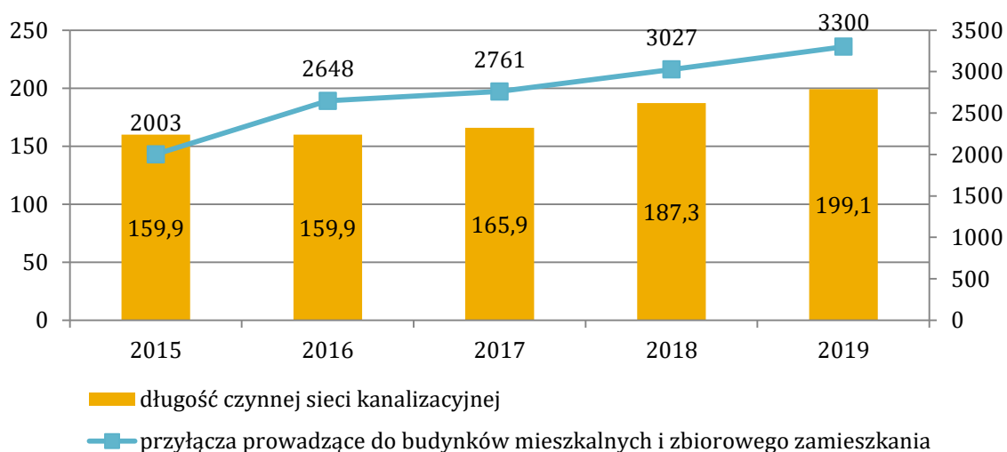
Wykres 18. Długość czynnej sieci kanalizacyjnej [km] i przyłączy w gminie Chełmiec w latach 2015-2019
