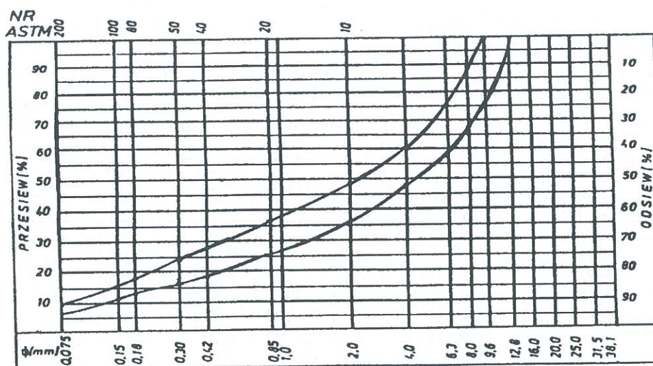
Rys. 6. Krzywe graniczne uziarnienia mieszanki mineralnej 0÷16 mm do warstwy ścieralnej z betonu
