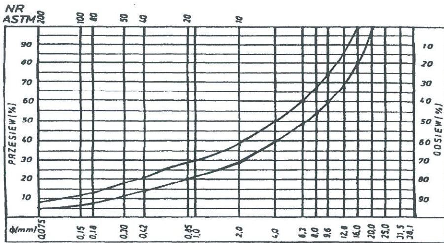
Rys. 4. Krzywe graniczne uziarnienia mieszanki mineralnej 0÷20 mm do warstwy ściernalnej z betonu asfaltowego dla KR 3-6
