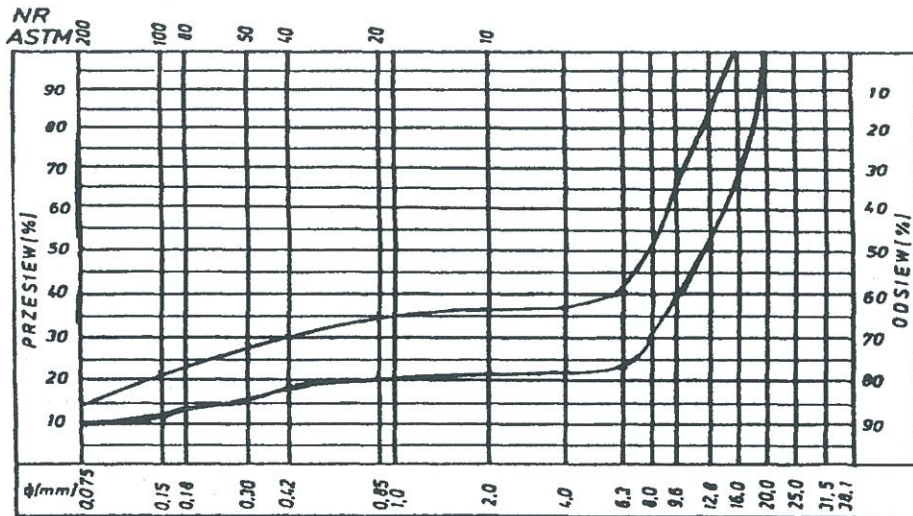
Rys. 5. Krzywe graniczne uziarnienia mieszanki mineralnej 0÷20 mm o nieciągłym uziarnieniu do warstwy ściernalnej z betonu asfaltowego dla KR 3-6
