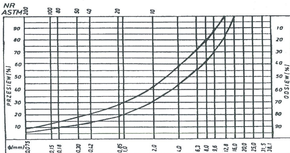
Rys. 5. Krzywe graniczne uziarnienia mieszanki mineralnej 0÷20 mm o nieciągłym uziarnieniu do warstwy ściernalnej z betonu asfaltowego dla KR 3-6
