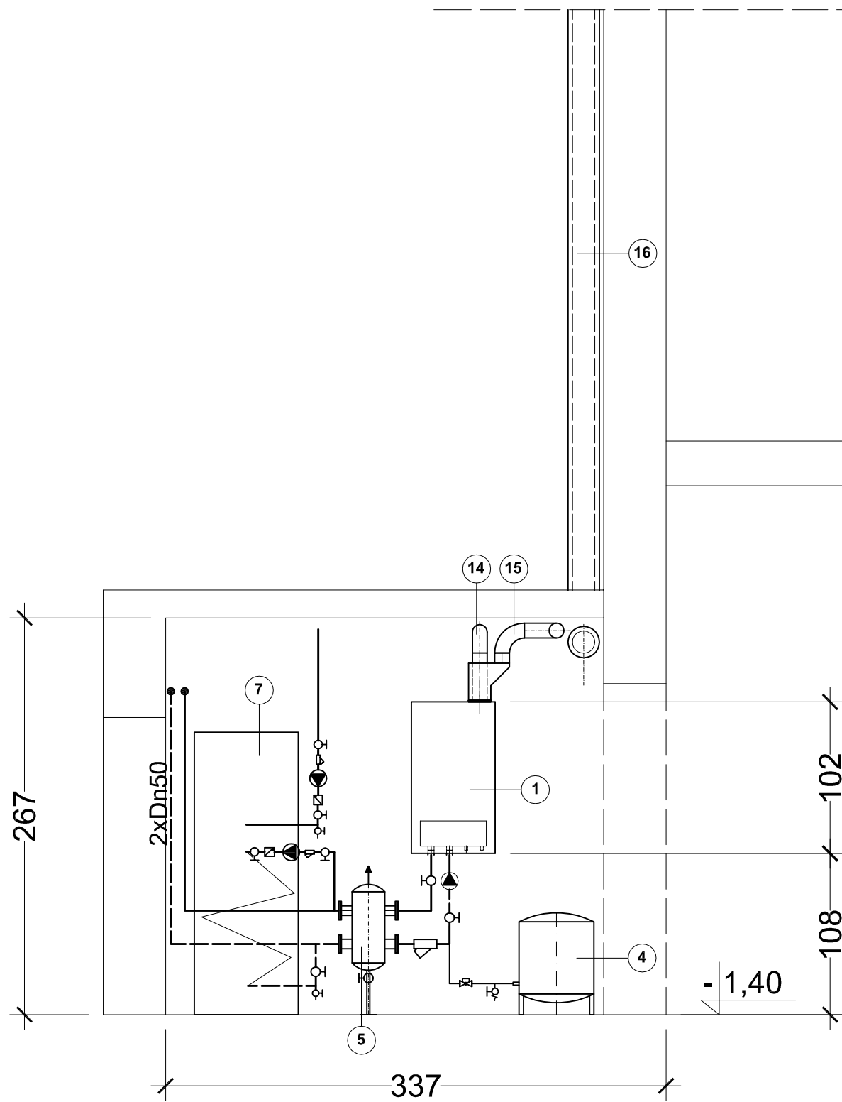
PRZEKRÓJ A-A
