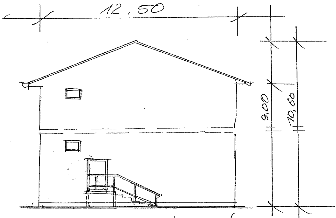
ELEWACJA POŁNOCNA OD STRONY PRYZALNI
